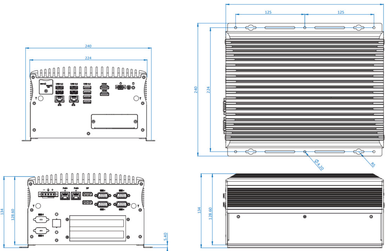
вид спереди
